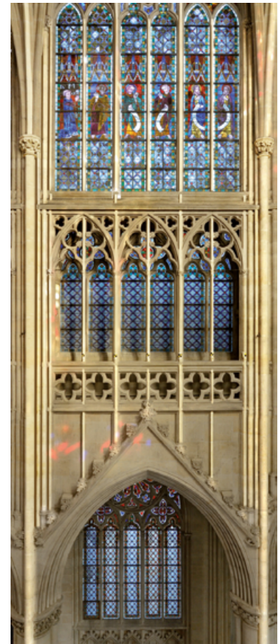
Le réseau de verticales part du galbe, traverse le triforium et monte jusqu'au sommet de la verrière haute rassemblant les différents étages.
