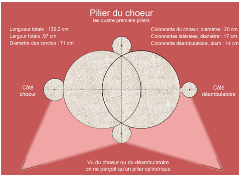
Schéma pilier chœur : Innovation de l'architecte du chœur, deux piliers encastrés de 71 cm de diamètre, pour donner l'illusion visuelle d'un seul pilier de 71 cm.
